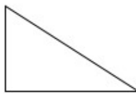
Hình tam giác vuông
