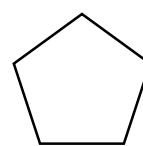
Hình ngũ giác đều
