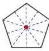
Hình ngũ giác đều có 5 trục đối xứng
