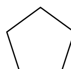
Hình ngũ giác đều
