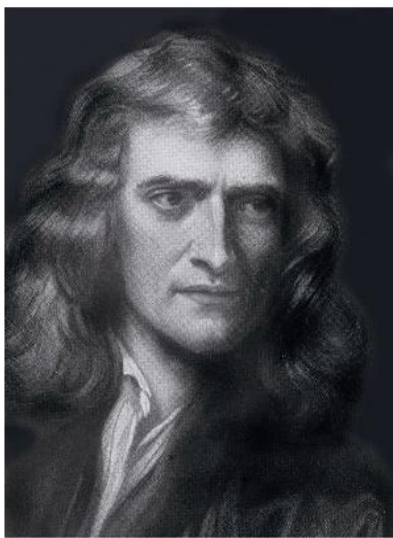
牛顿
