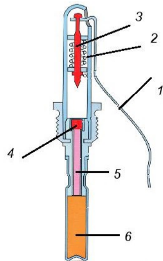
Hình 6-3. Cấu tạo bộ phận gây nổ lựu đạn Φ1
