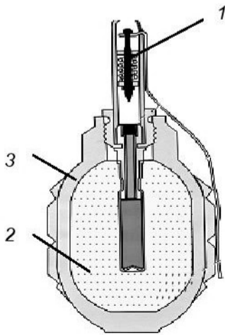
Hình 6-2. Cấu tạo lựu đạn Φ1
