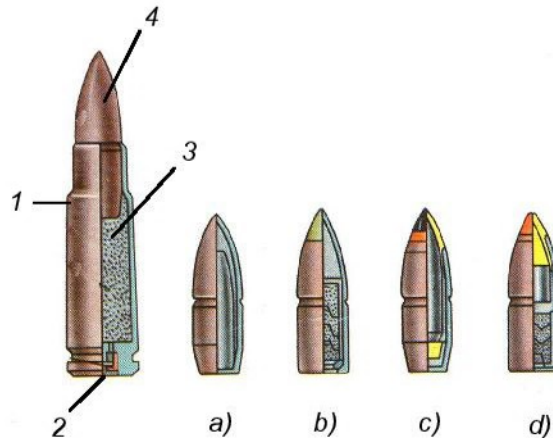
Hình 4-17. Đạn K56
