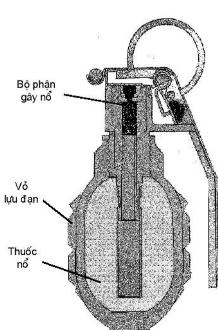
Hình 6-4. Cấu tạo lựu đạn cân 97
