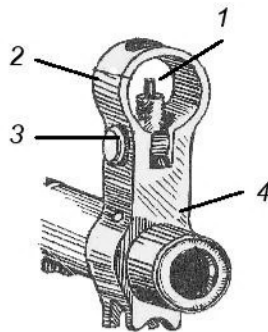
Hình 4-32. Đầu ngắm
