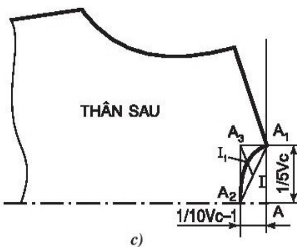
Hình 46b, c. Cách vẽ cổ tròn cơ bản
