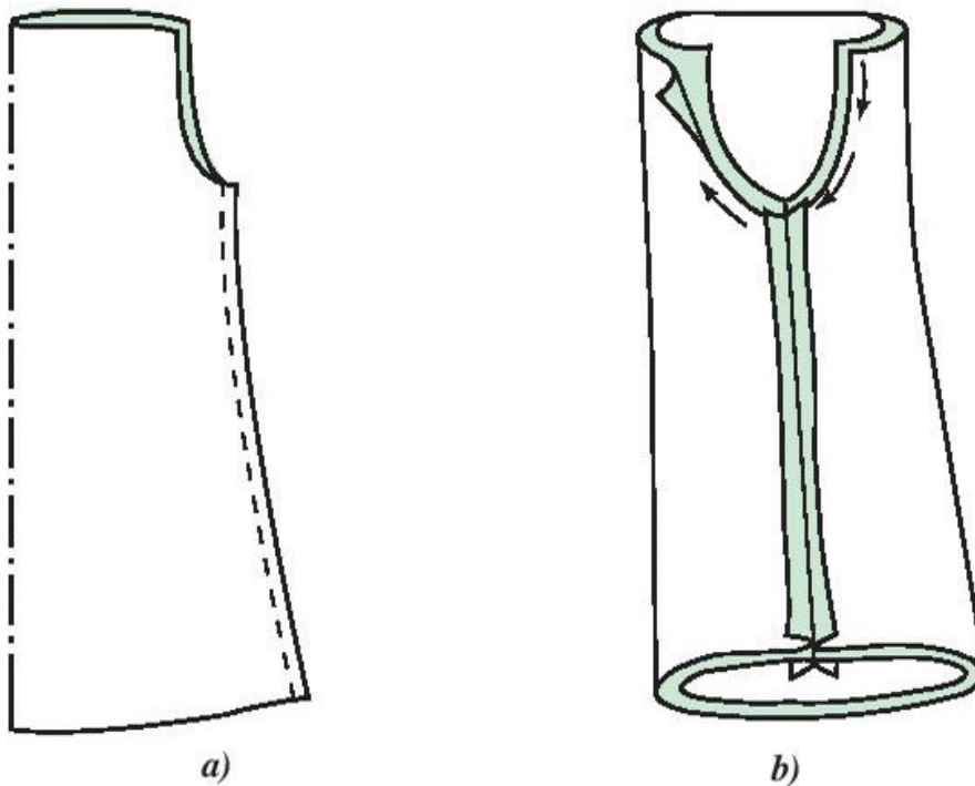
Hình 40. Cách may quần dài
