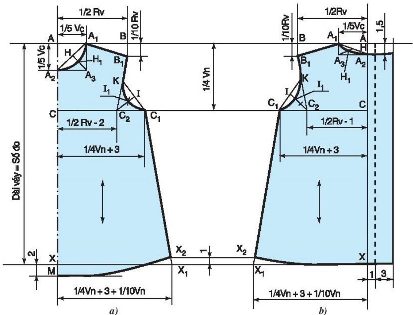
Hình 34. Bản vẽ cắt may váy em gái kiểu liền thân : a) Thân trước ; b) Thân sau.
