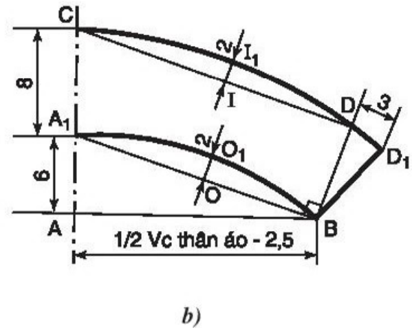
Hình 51. Cách vẽ bâu lá sen đứng
