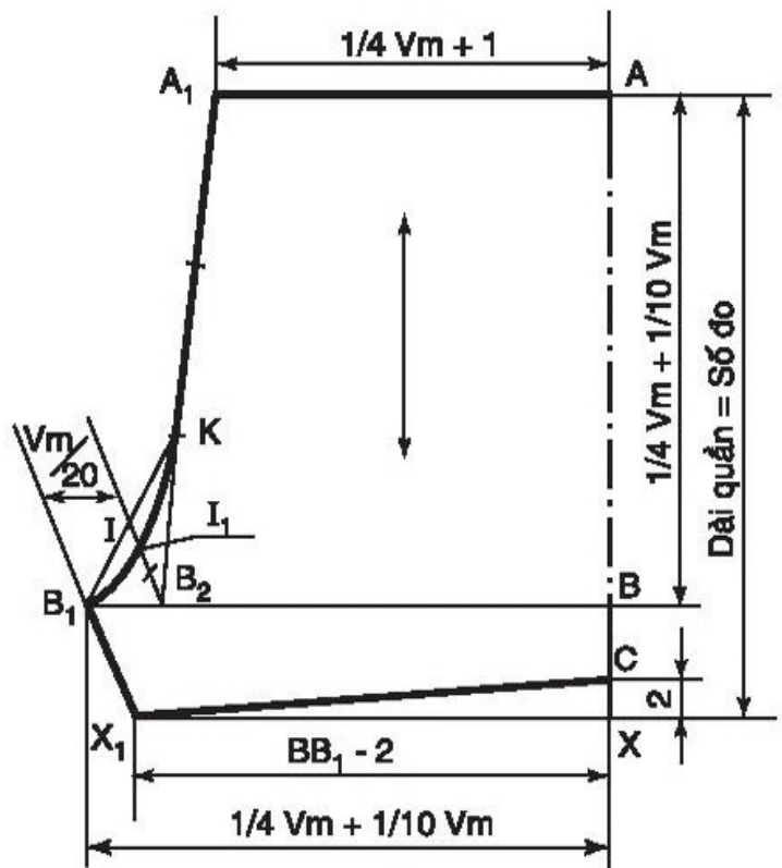
Hình 35. Bản vẽ quần đùi
