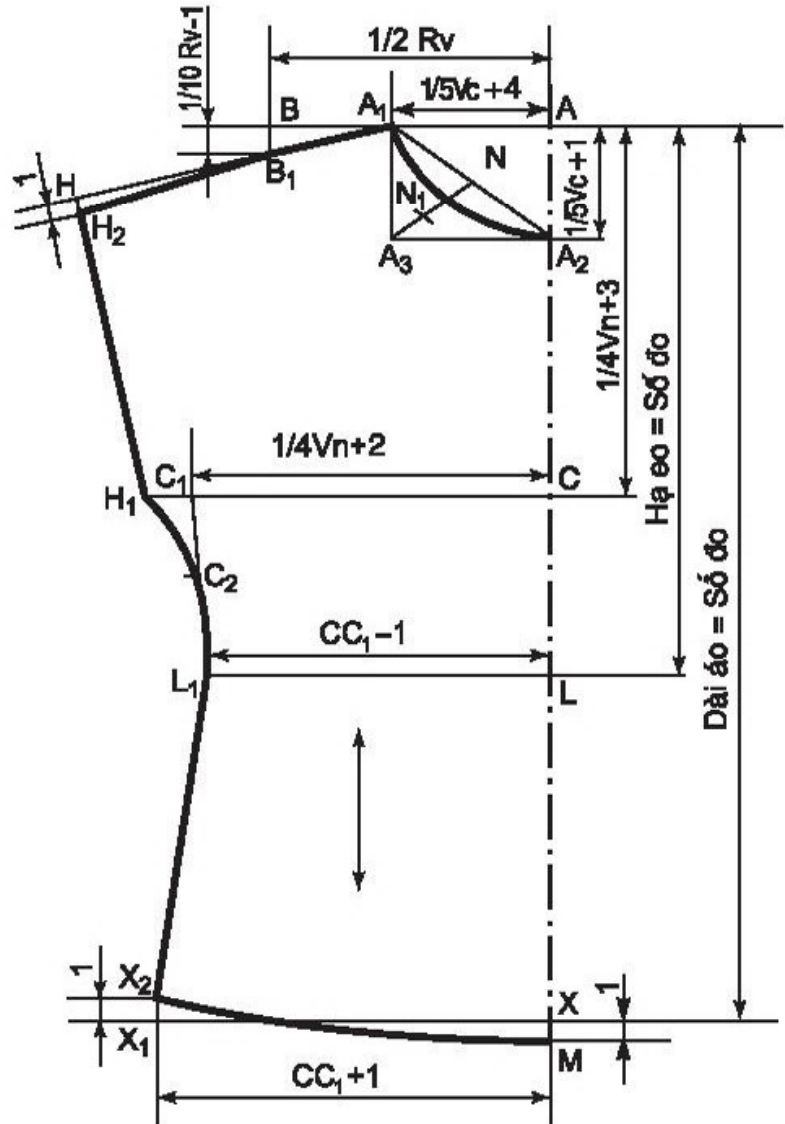
Hình 43. Bản vẽ thân trước
