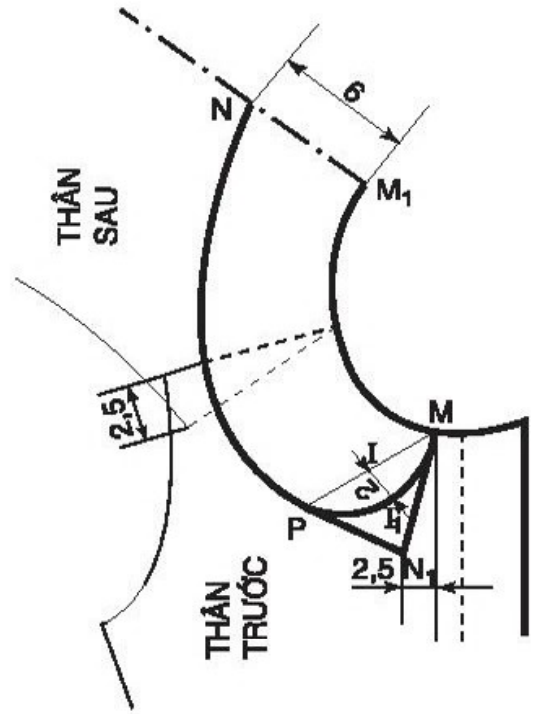
Hình 52. Cách vẽ bâu lá sen nằm
