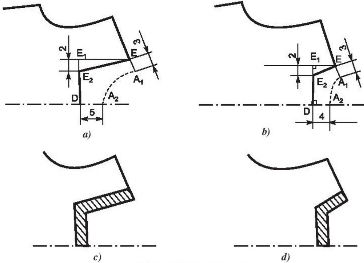
Hình 48. Cách vẽ cổ vuông : a) Thân trước ; b) Thân sau ; c) Vải viền cổ thân trước ; d) Vải viền cổ thân sau.
