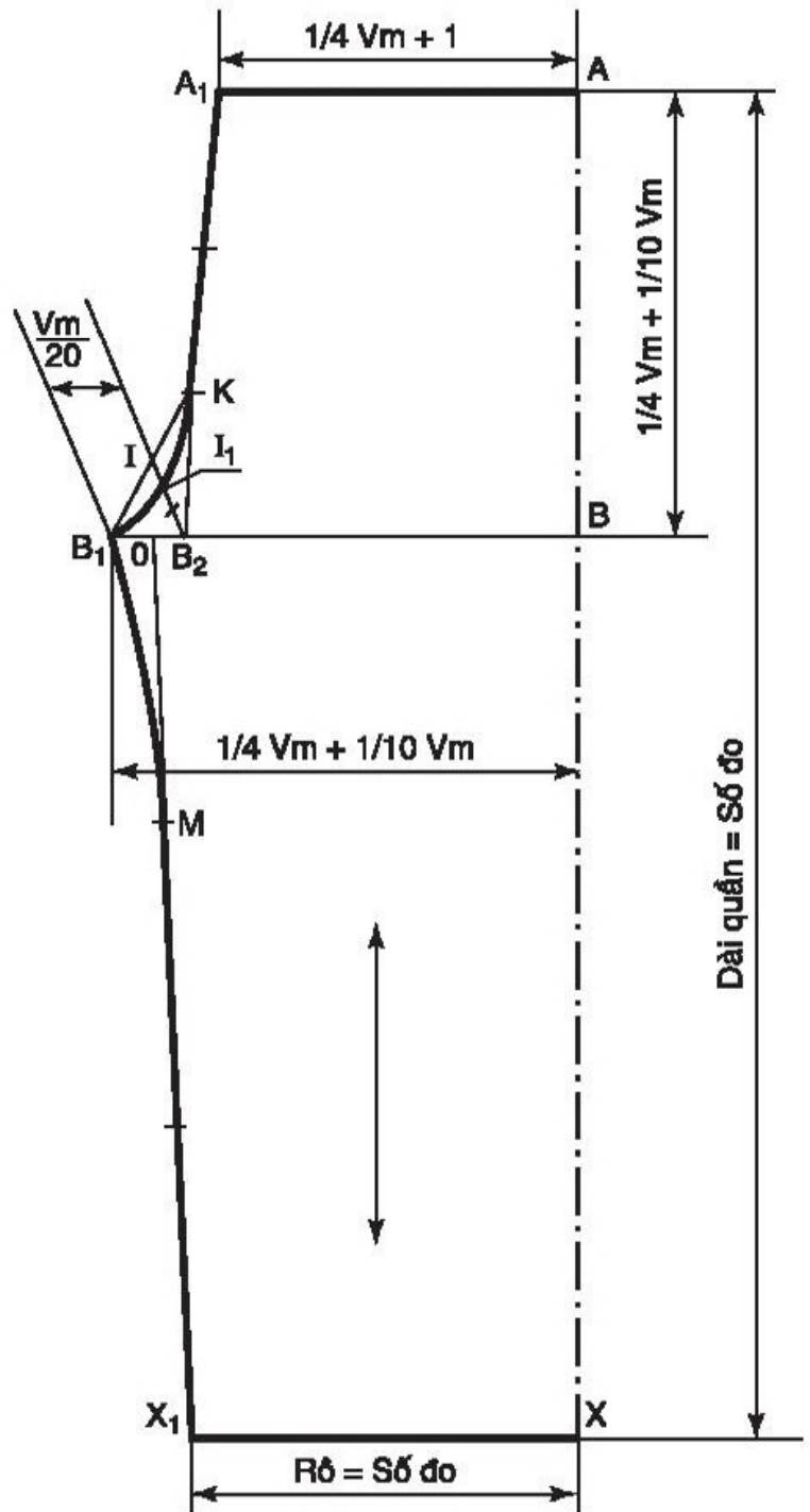
Hình 38. Bản vẽ quần dài (ống thẳng)
