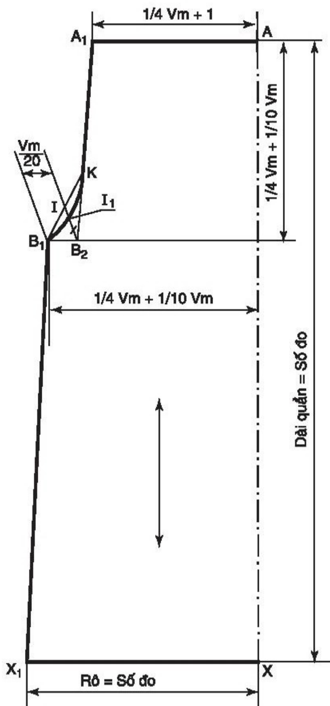
Hình 39. Bản vẽ quần dài (ống rộng)
