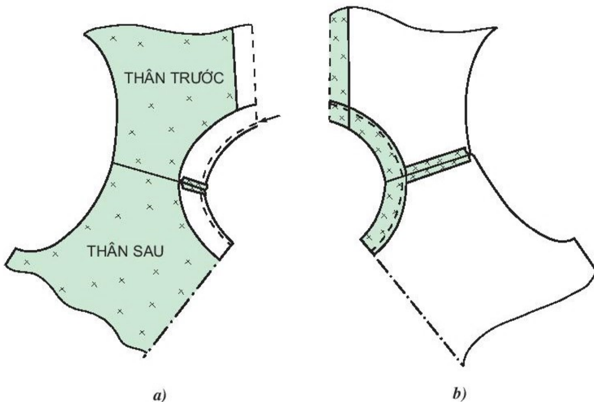
Hình 50. Cách may cổ tròn
