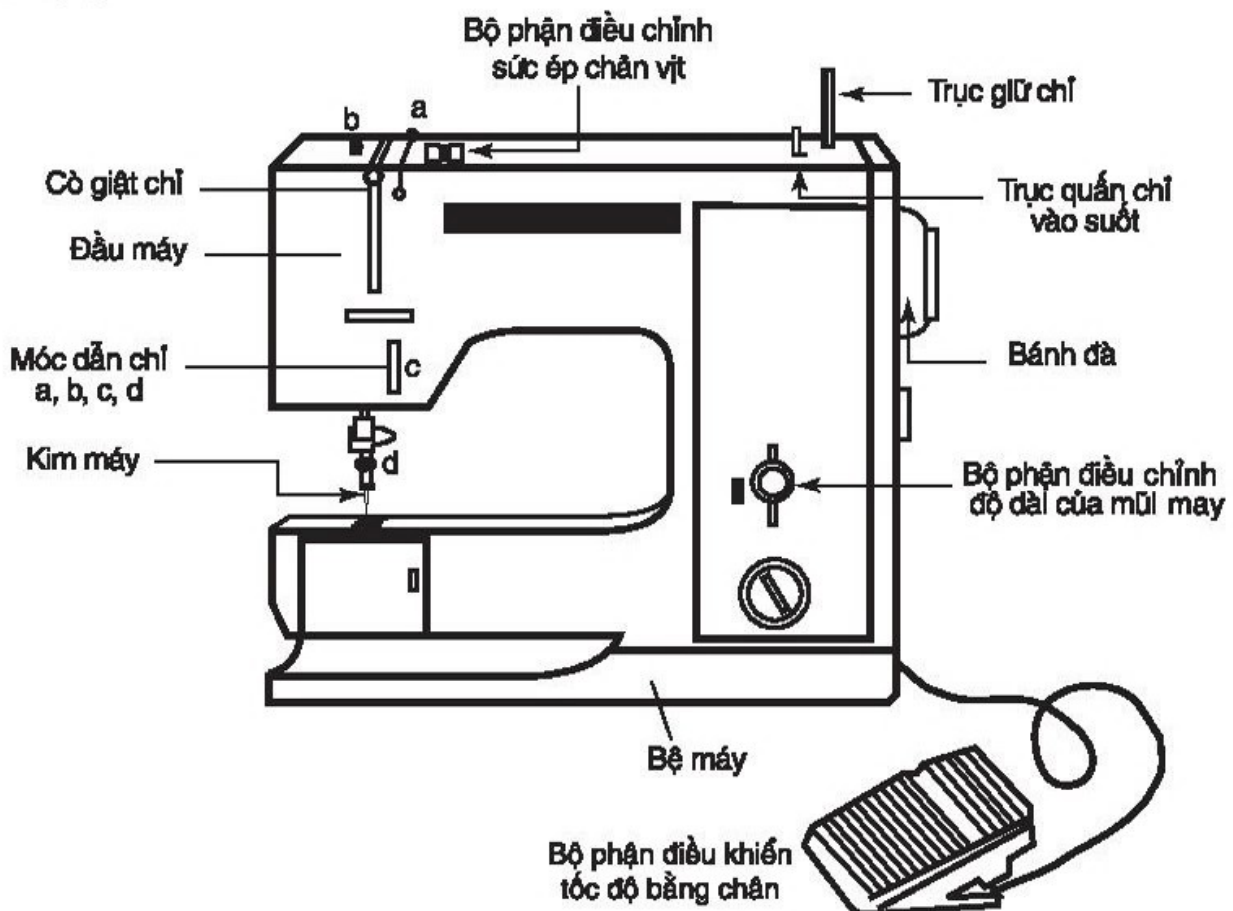
Hình 11. Máy may chạy điện
