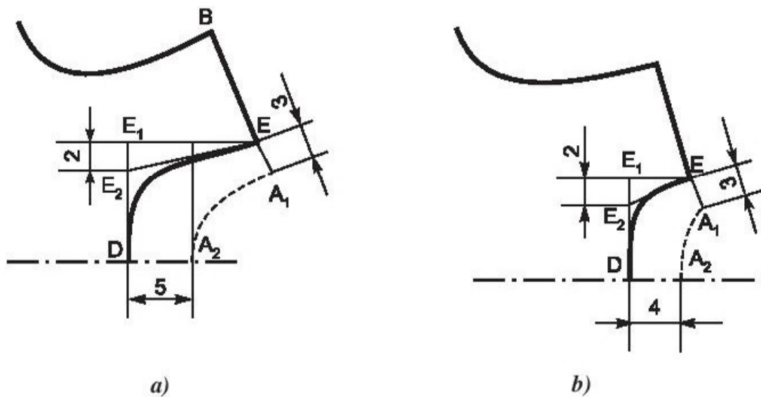
Hình 49. Cách vẽ cổ chữ U
