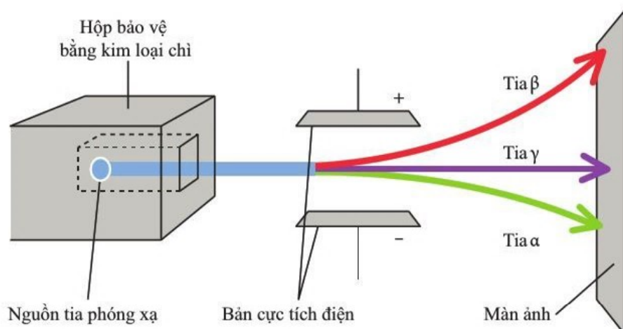
Hình 2.1. Thí nghiệm nghiên cứu thành phần tia bức xạ
