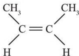
cis -2-butene
