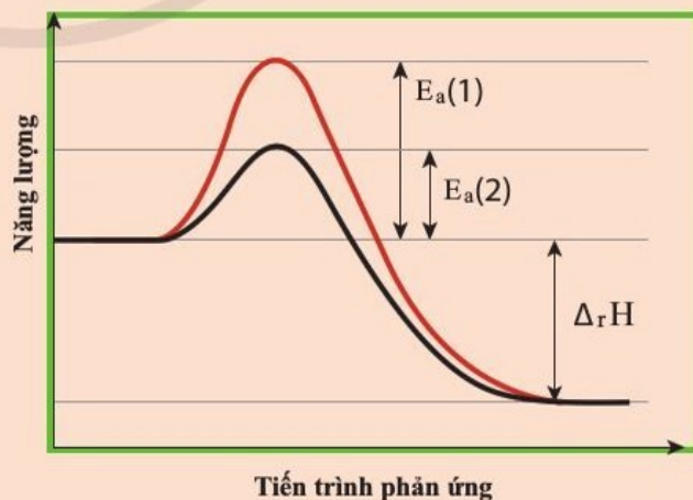
Hình 3.3. Đồ thị biểu diễn các mức năng lượng hoạt hoá khác nhau của phản ứng
