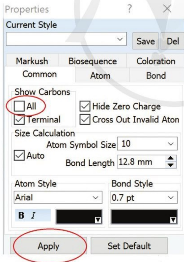
Hình 8.2. Cửa sổ Properties
