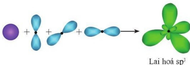
Hình 1.2. Sự hình thành các dạng lai hoá sp , sp^2 và sp^3
