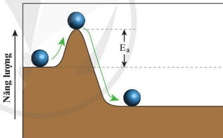
Hình 3.1. “Hòn bi hoá học” và hàng rào năng lượng E_a
