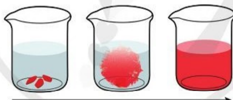
Hình 4.3. Quá trình hoà tan tinh thể potassium dichromate vào nước
