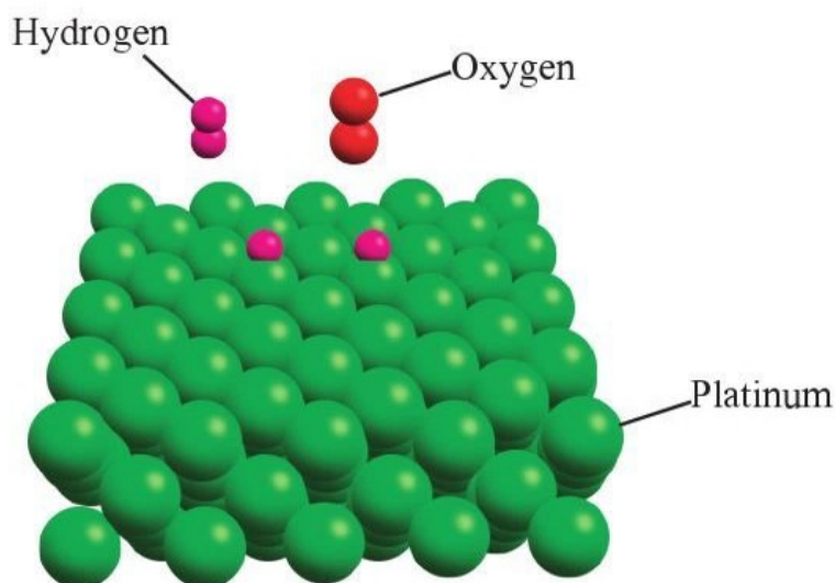
Hình 3.4. Phân tử H_2 bị phá vỡ liên kết trên bề mặt chất xúc tác Pt
