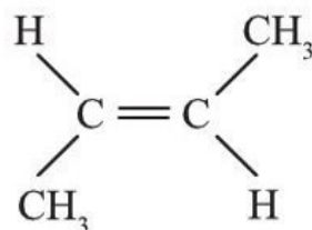
trans -2-butene
