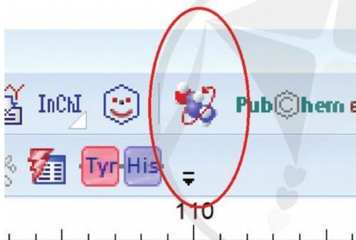
Hình 8.3. Vị trí nút 3D Viewer
