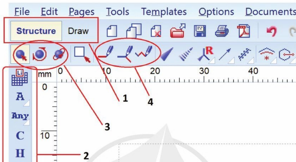
Hình 8.1. Cửa sổ ChemSketch
