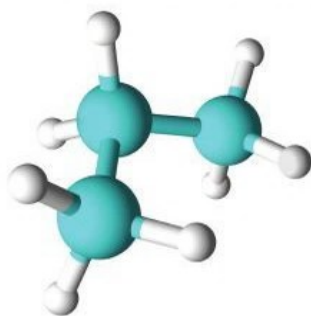
Hình 8.4. Hình ảnh cấu trúc 3D của propane
