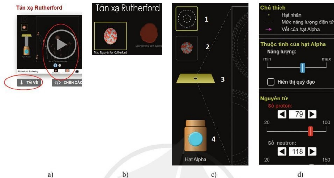
Hình 9.1. Thí nghiệm lá vàng của Rutherford
